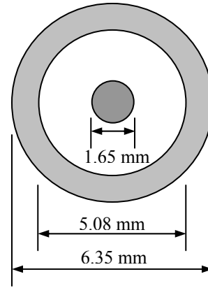
(b) Dimensions
